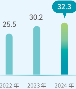
拉斯邦巴斯矿山铜精矿含铜产量 单位：万吨
